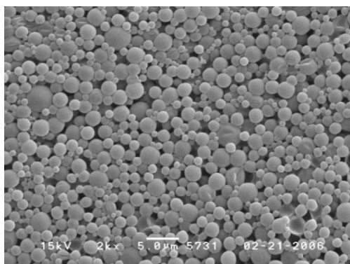
パラフィン系樹脂が入ったマイクロカプセル (マイクロカプセルの粒径は1.0～5.0μで、平均3.0μ)
